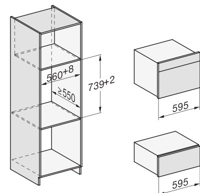
Einbau im Hochschrank mit 45er B/BM/DG/DGM/DGC/CVA/M
