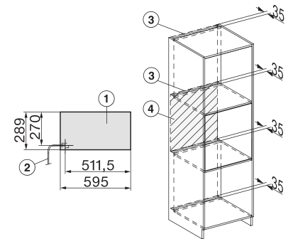
Einbau im Hochschrank
