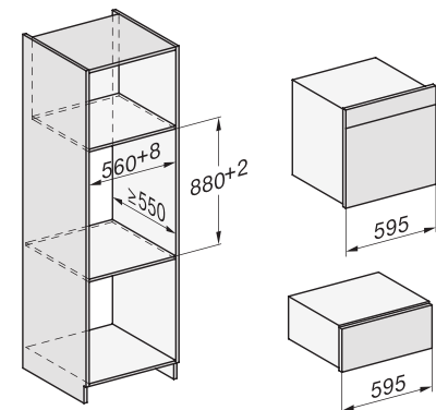
Einbau im Hochschrank mit 60er B/DO/DGC
